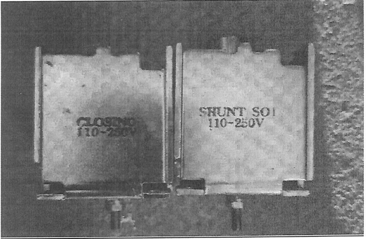
Fotoğraf 3. Motorlu Transfer Şalterine Ait Kapama Bobini ve Açma Bobini Görseli
