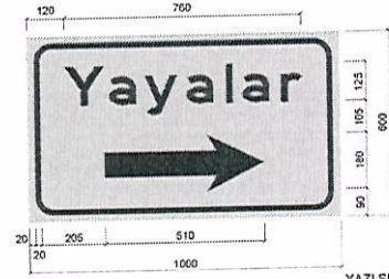
(YB-3) YAYA YÖNLENDİRME LEVHASI
