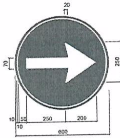
(TT-35a) SAĞA MECBURİ YÖN
