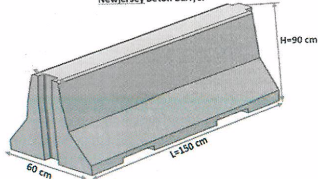
Karayolları Standartlarında Newjersey Beton Bariyer
