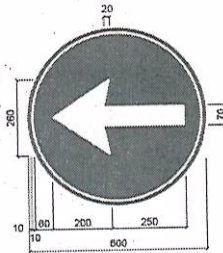
(TT-35b) SOLA MECBURİ YÖN
