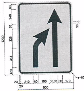
(YB-4a) ŞERİT DÜZENLEME LEVHALARI
